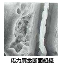
応力腐食断面組織
