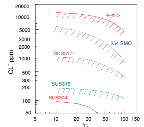
●塩素イオン 環境でのプレート板材の使用限界
