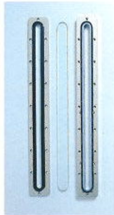
液面計パッキン (サイズ600L用)
