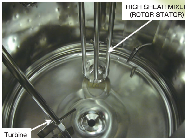
TurbineとHIGH SHEAR MIXERの2軸攪拌槽の内部
